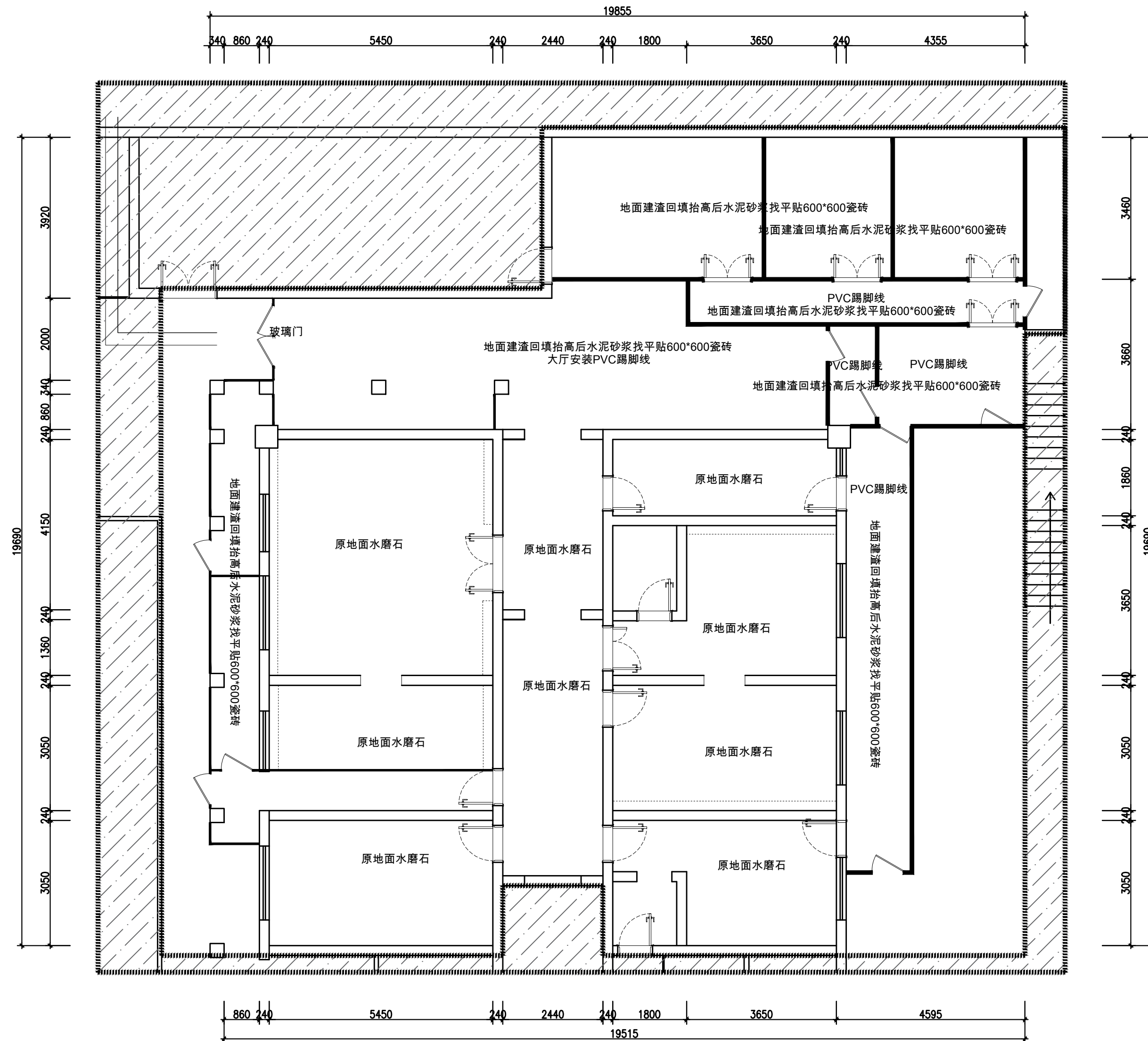
地面布置图 SCALE:1/70
